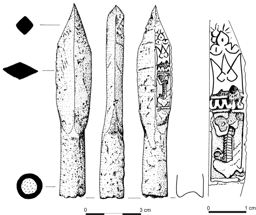
Рис. 7. Прикрашений наконечник болта від арбалета з Кросна (за Kotowicz P. N. Muzyczuk A. Militaria średniowieczne... , rys. 7).
