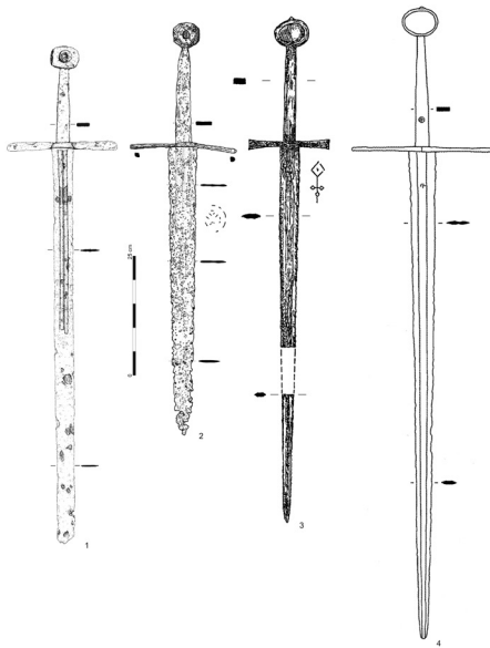
Рис. 9. Пізньосередньовічні мечі, виявлені на території Червоної Русі: с. Динів (1), околиця Яслицьк (2), Радимно (3-4) (1 – за Glinianowicz M., Kotowicz P. N. Dwa nieznane... , рис. 1:b; 2 – за Kotowicz P. N., Glinianowicz M. Późnośredniowieczny miecz... , рис. 1:1; 3 – за Koperski A. Miecz średniowieczny... , рис. 1; 4 – за Biborski M., Żabiński G. Two Late Medieval Swords... , Fig. 3:b).
