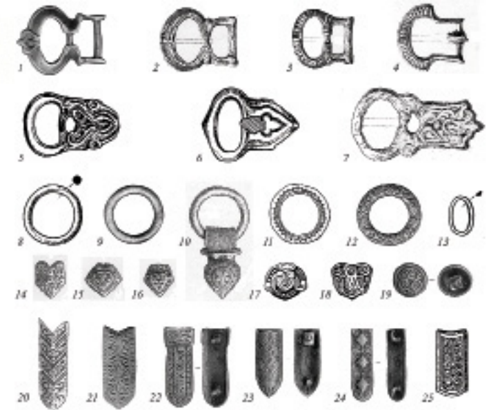
Рис. 2. Детали поясной гарнитуры: 1–7 – пряжки (1–4 – лировидные, 5–7 – щитковые); 8–12 – поясные кольца; 13 – кольцо-скобка; 14–19 – бляшки-накладки; 20–25 – ременные наконечники. 1–9, 11–25 – бронза, 10 – бронза, кожа. Источники: 1. Соболев, Торопов 2010. Рис. 1, 1; 2. Спицын 1896. Табл. VII, 5; 3. Спицын 1896. Табл. VII, 7; 4. Спицын 1896. Табл. XV, 5; 5. Михайлов, Соболев 2000. Рис. 2, 1; 6. Фоянков 1986; 7. Спицын 1896. Табл. VII, 2; 8. Михайлов, Соболев 2000. Рис. 2, 9; 9. Соболев, Торопов 2010. Рис. 1, 19; 10. Спицын 1896. Табл. XVI, 19; 11. Курганная группа Березицы III, курган 2 погр. 2; 12. Соболев, Торопов 2010. Рис. 1, 17; 13. Михайлов, Соболев 2000. Рис. 2, 8; 14. Спицын 1896. Табл. XVI, 2; 15. Спицын 1896. Табл. XVI, 4; 16. Спицын 1896. Табл. XVI, 1; 17. Михайлов, Соболев 2000. Рис. 2, 6; 18. Михайлов, Соболев 2000. Рис. 2, 5; 19. Соболев, Торопов 2010. Рис. 1, 2; 20. Спицын 1896. Табл. XVI, 5; 21. Бранденбург 1895. Табл. VI, 12; 22. Соболев, Торопов 2010. Рис. 1, 13; 23. Соболев, Торопов 2010. Рис. 1, 14; 24. Соболев, Торопов 2010. Рис. 1, 15; 25. Михайлов, Соболев 2000. Рис. 2, 10.
